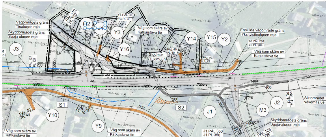
Kuva 11. Ote Vassor-Öliksen tiesuunnitelmasta. © Destia
