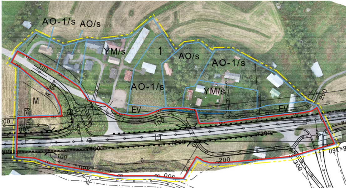
Kuva 23. Ote kaavaehdotuksen teknisestä tarkistuksesta tiesuunnitelma ja ilmakuva taustana.
