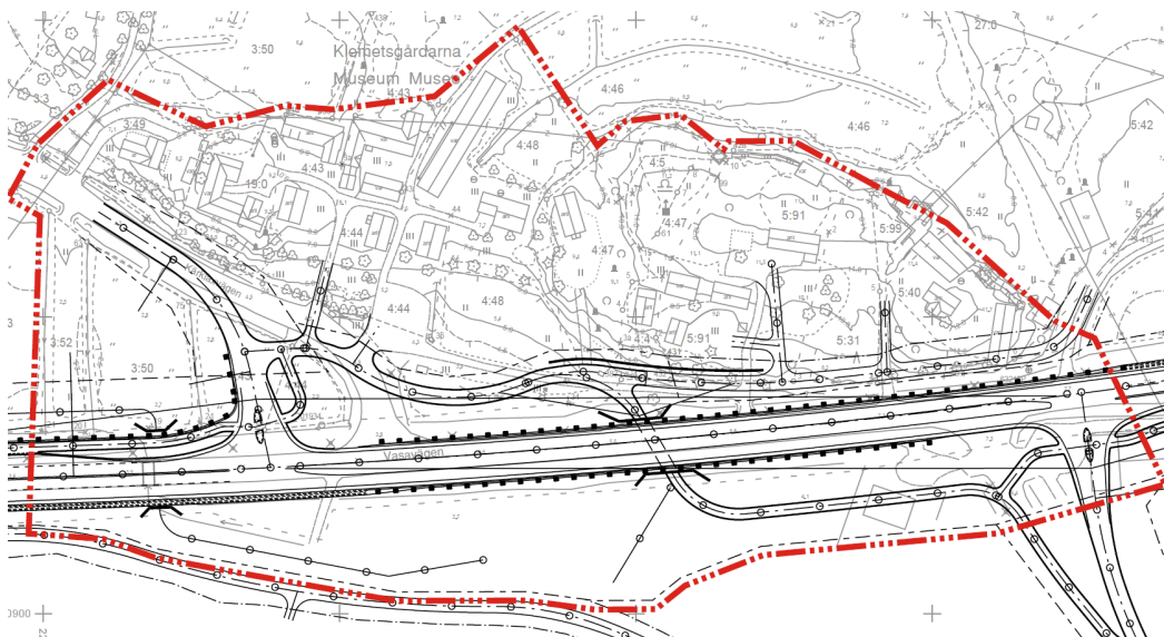
Kuva 12. Tiesuunnitelman ratkaisuja, suunnittelualan likimääräinen rajaus osoitetaan punaisella.
